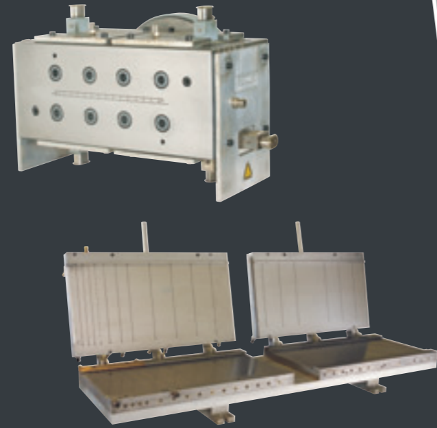
Kalibreereenheid voor 250 mm vlakpaneel ↑ Unité de calibration pour panneaux lisses de 250 mm ↑ Calibrator for 250 mm flush panels ↑
